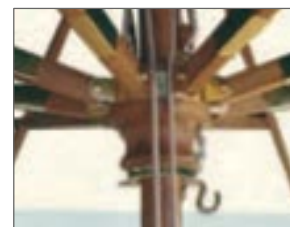
ANELLO DI RINFORZO E U-BRACKETS (STECHE SOSTITUIBILI SINGOLARMENTE) RING AND U-BRACKETS (SPOKES CAN BE REPLACED SINGULARLY)
